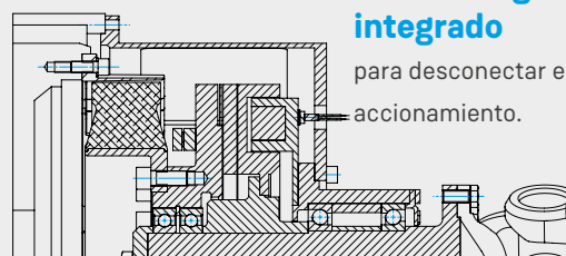
Tipo AC...F2 con acoplamiento electromagnético
