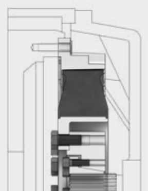
Tipo AC...F2 con casquillo de sujeción dentado
